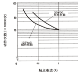
电气寿命曲线
